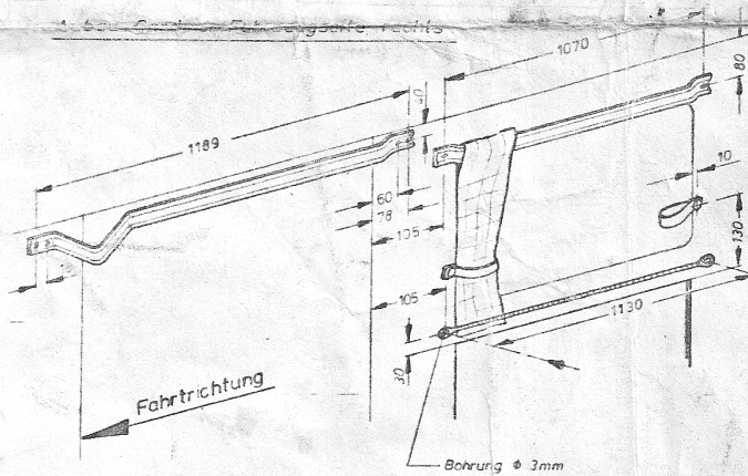
Anbau Gardinen Fahrzeugseite links:
