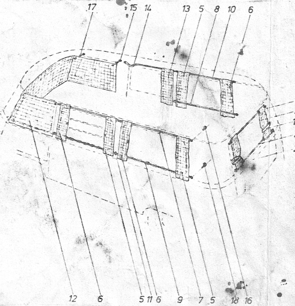
Anbau Gardinen Heckklappe
