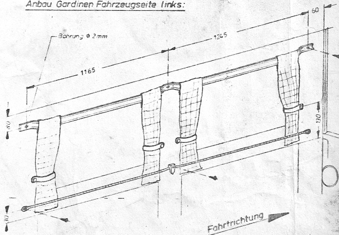
Anbau Gardinen Fahrzeugseite links:
